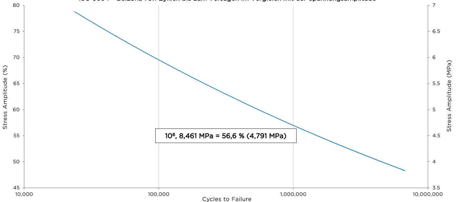
ISO 9664 - Belzona 7311 Zyklen bis zum Versagen im Vergleich mit der Spannungsamplitude
